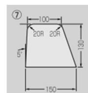
【成形断面参考図】
